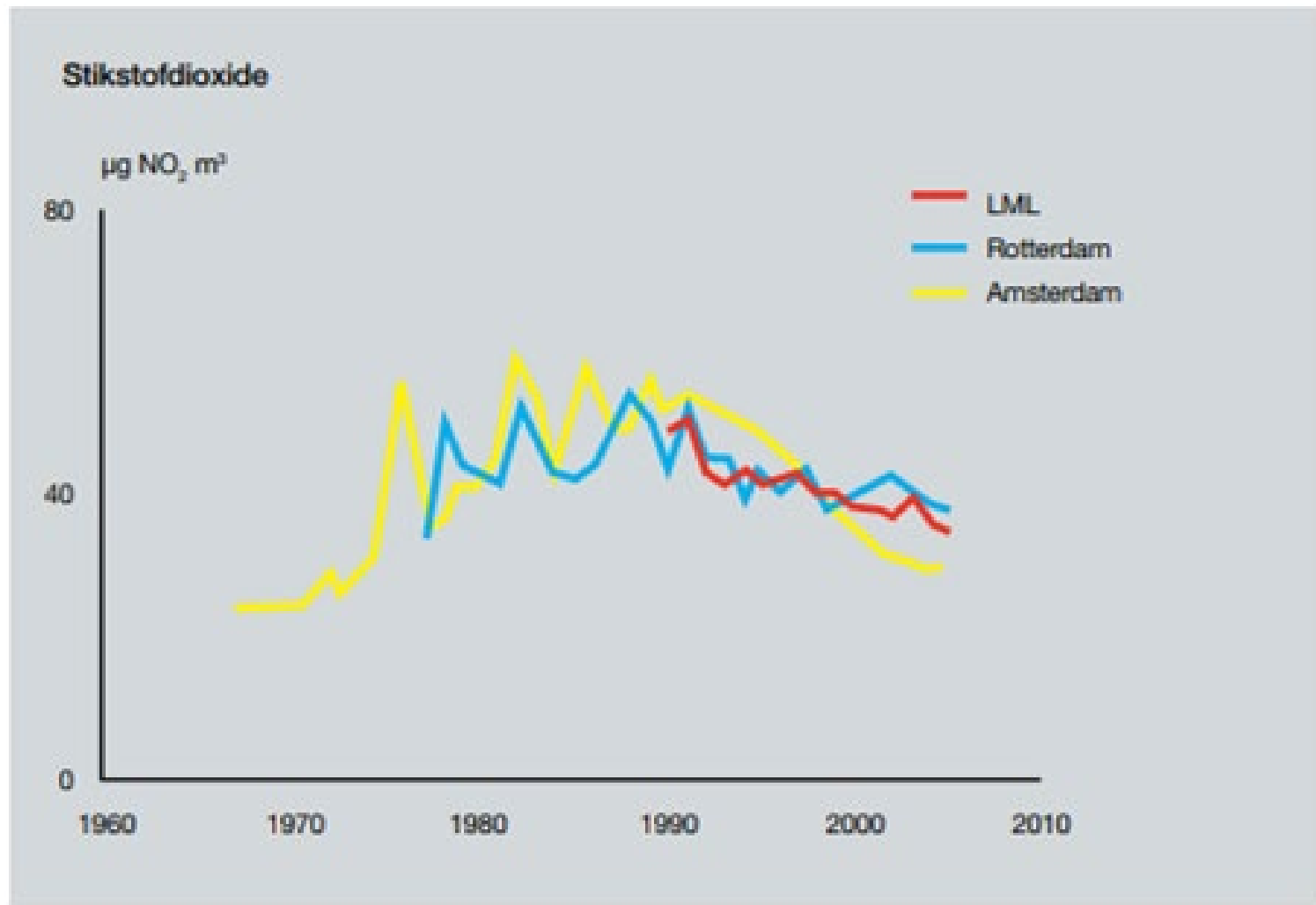
Figuur 6: Ontwikkeling van de stedelijke luchtkwaliteit voor stikstofdioxide ( \text{NO}_2 ). De gestippelde lijnen geven de meetresultaten van individuele stations. De zwarte lijn ("LML") geeft het gemiddelde van de stations in de stadsachtergrond in het Landelijk Meetnet Luchtkwaliteit.
